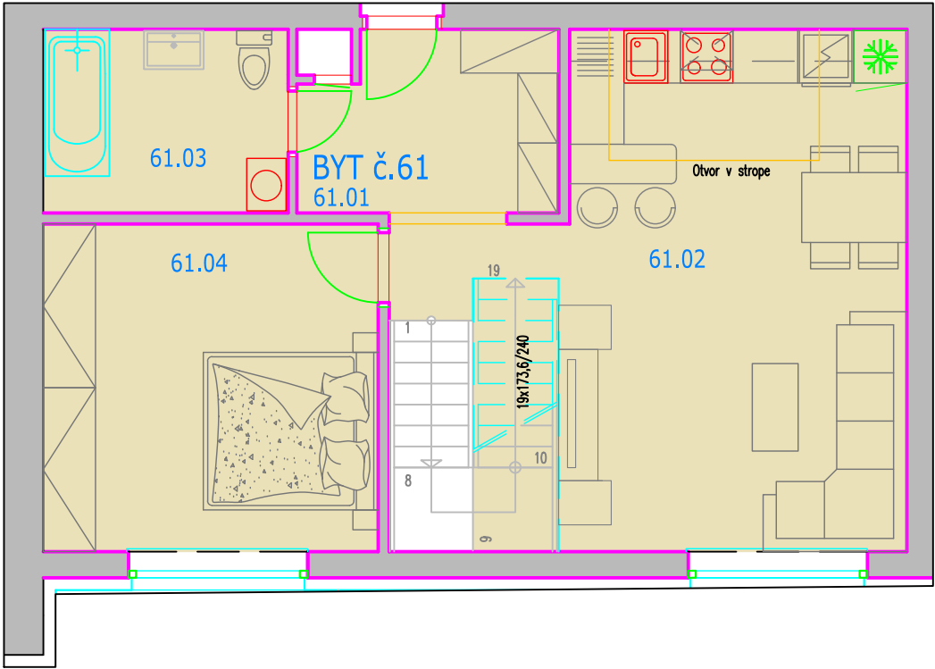
PÔDORYS 4.NP - BYT č. 61 (MEZONET)
