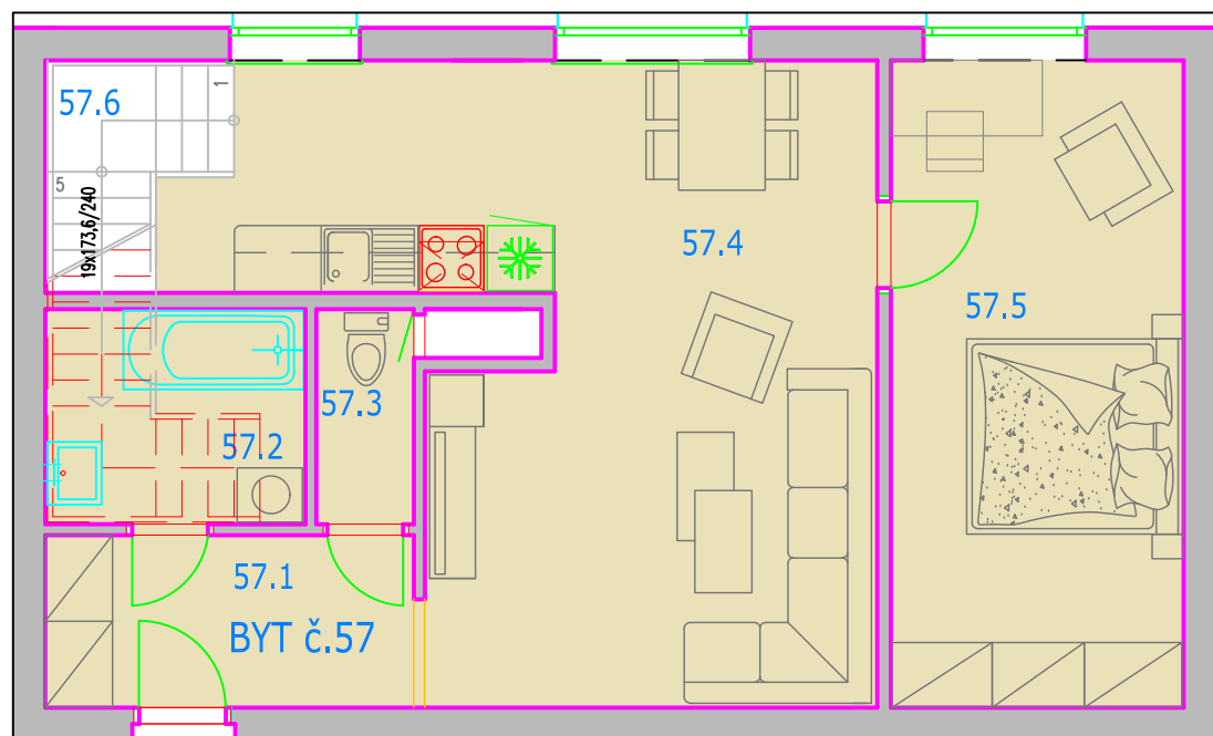
PÔDORYS 4.NP - BYT č. 57 (MEZONET)
